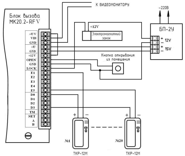
Рис. 2 Пример монтажа блока вызова МК20.2-RFV
